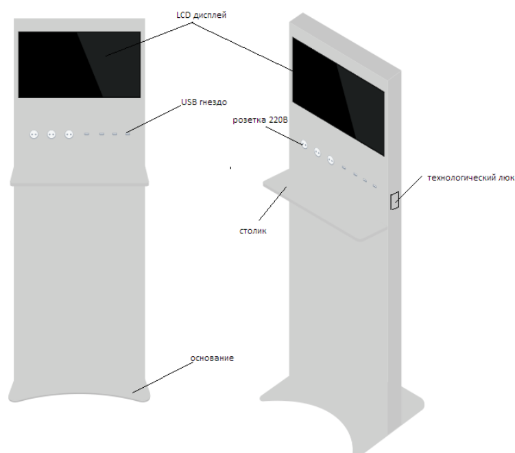
Рис.1 Общий вид автомата
